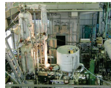
(写真：熱工学実験棟，高密度除熱強制対流実験設備)
